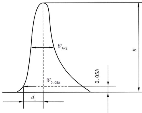
图 A.2 拖尾因子(T)示意图
