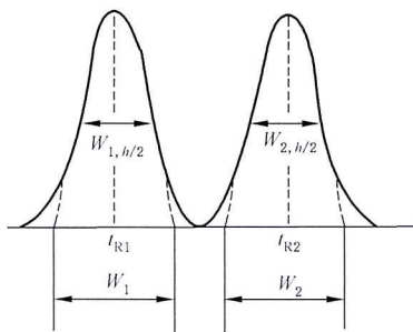
图 A.1 分离度(R)示意图
