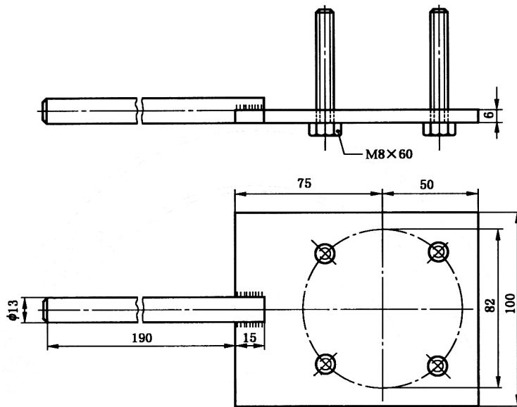
图 7 试验槽支架
