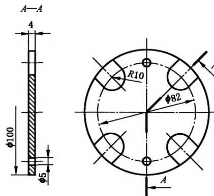
图 10 透明盖(可选)
