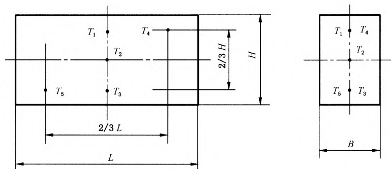
图 1 L 不小于 0.7\text{ m} 顶开式冷藏箱的温度测量点
