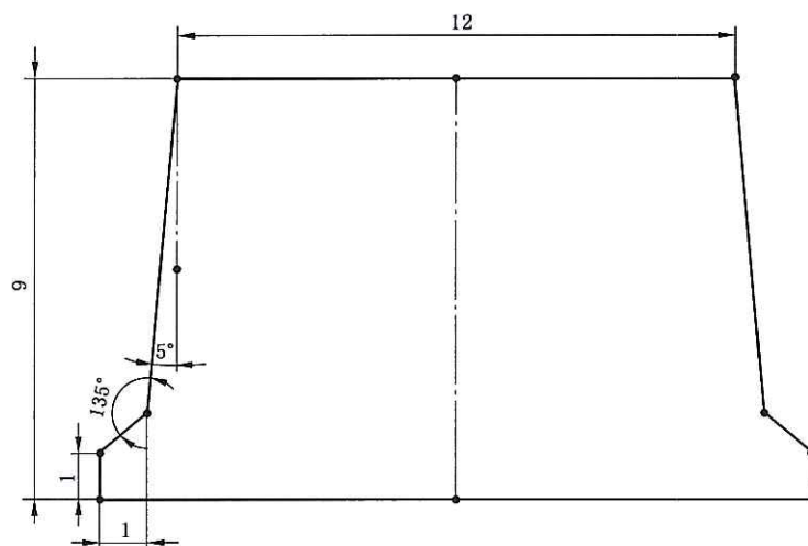
图 A.1 标准预备体模型尺寸
